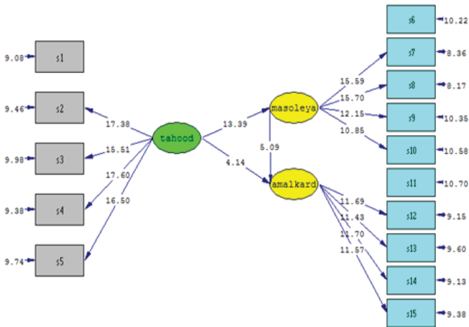
شکل ۳: نمودار محاسبات آماره تی
