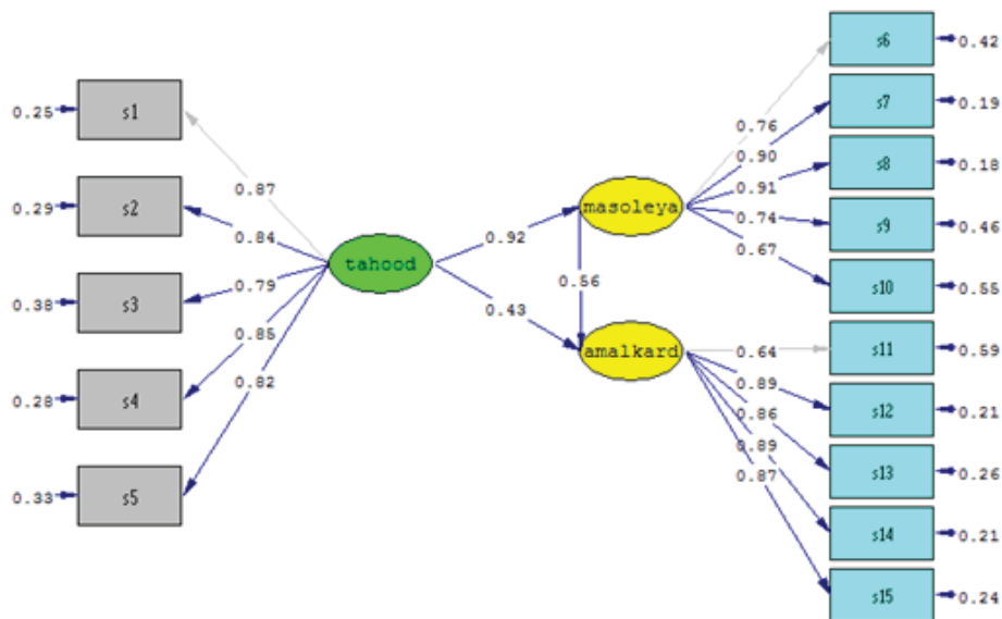
شکل ۲: نمودار معادلات ساختاری بر اساس مقادیر استاندارد
