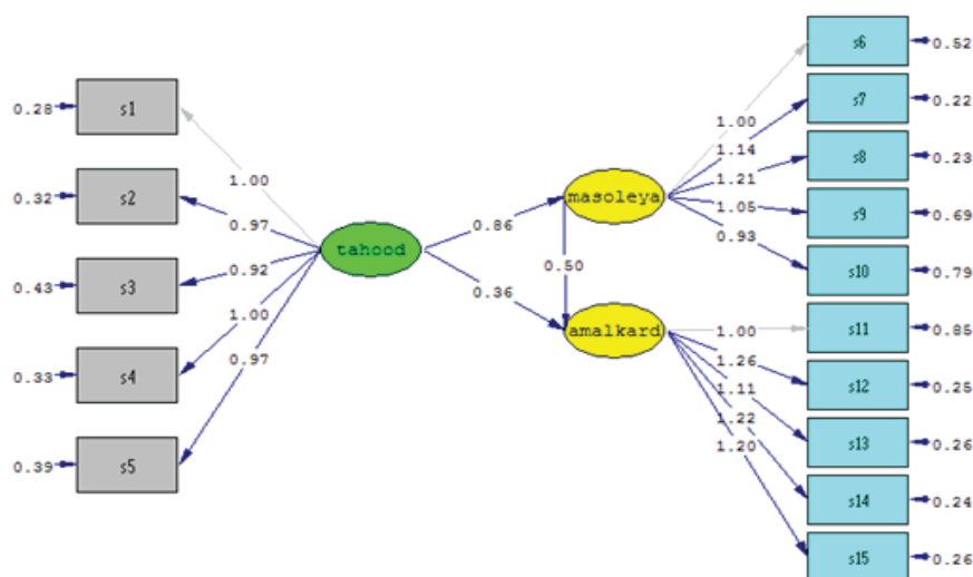
شکل ۱- نمودار معادلات ساختاری بر اساس مقادیر تخمین زده شده
